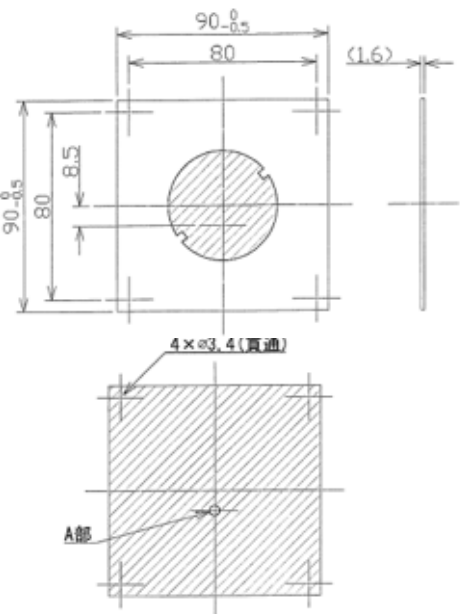
レクテナ用アンテナ素子
