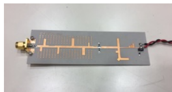
レクテナ用整流器
