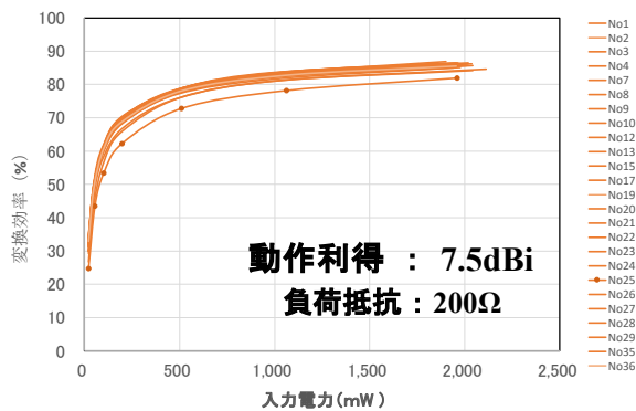
第 5 図 37 素子レクテナアレイユニット
