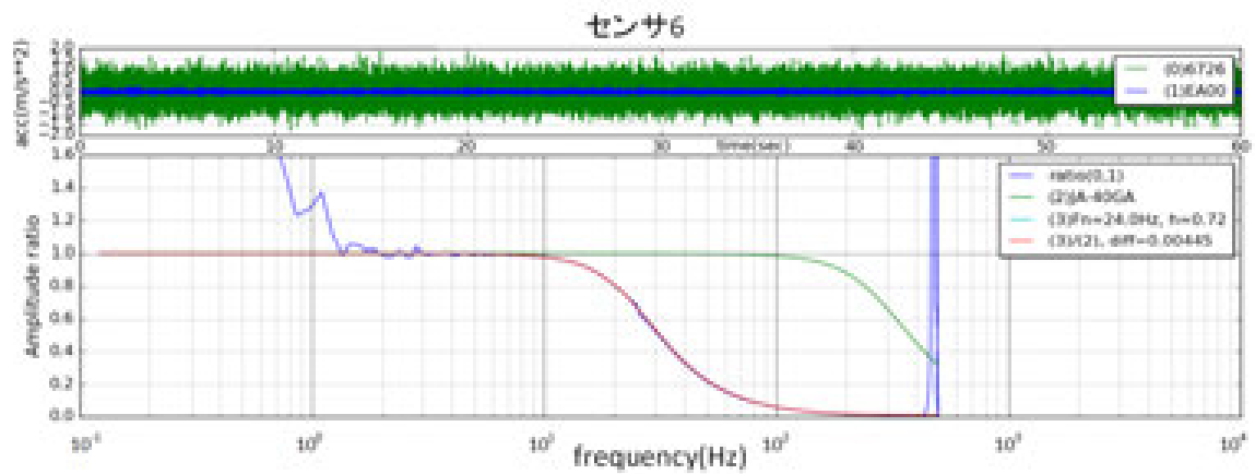
図4 光センサの検証結果
