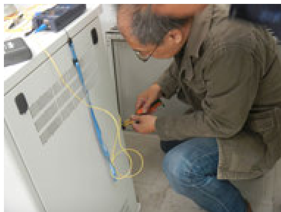
写真 6 光ケーブル空き芯線の通信テスト
