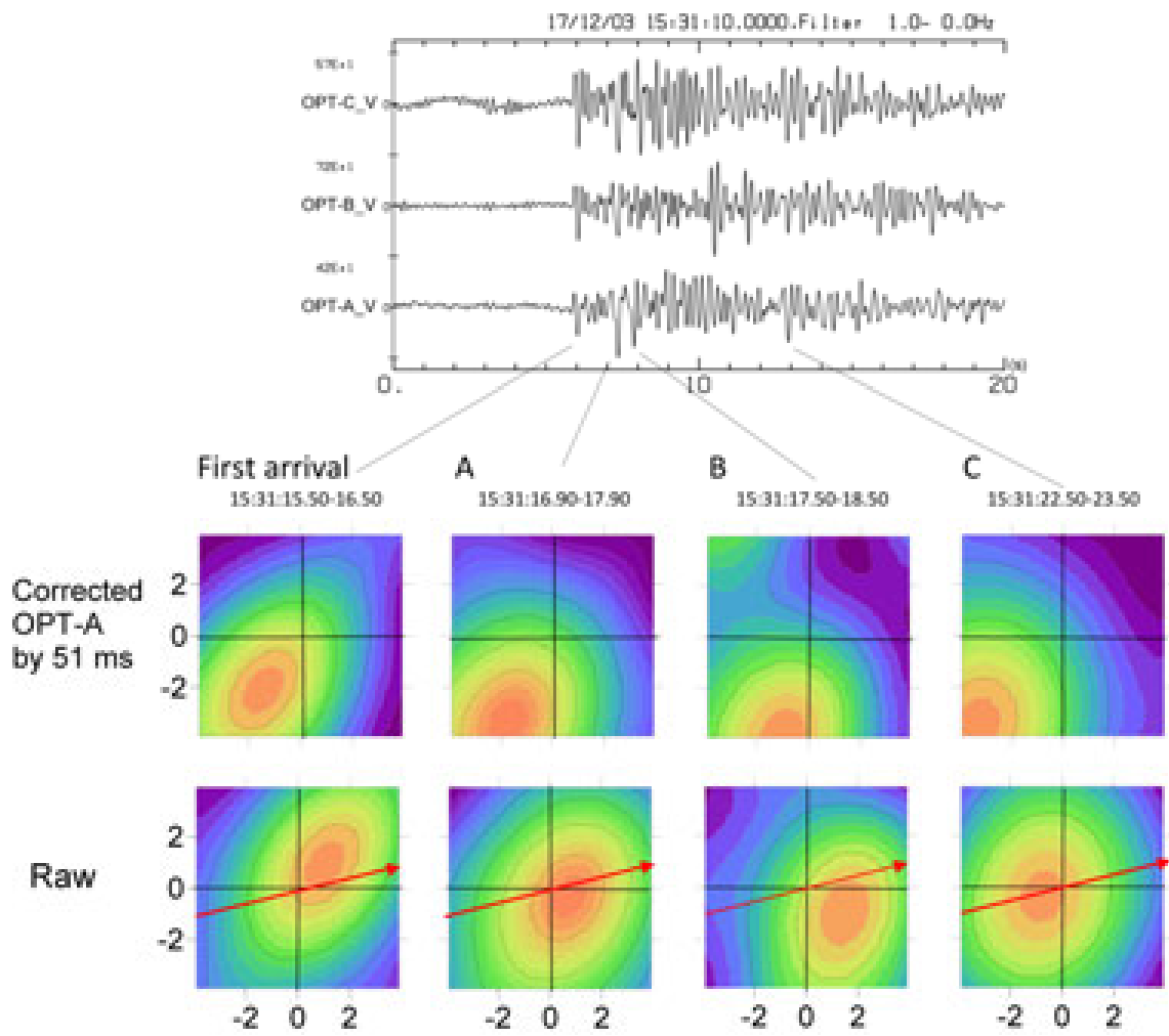
浅部構造にもとづく走時補正による火山性地震の地震波到来方向の補正. 最下段 RAW は走時補正を施さない場合の結果, その上は走時補正を施した結果を示す.
